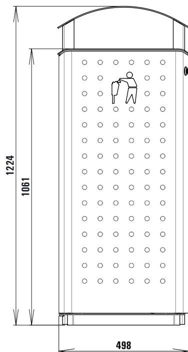
Vooraanzicht
