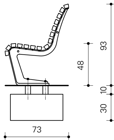
Zijaanzicht
